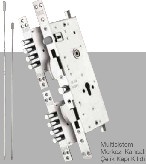
Kancalı Çelik Kapı Gömme Kilidi
